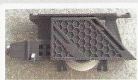
Roulement bas à billes 4 ergots anti-déraillement
